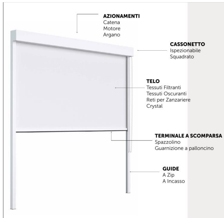
I componenti della tenda a rullo da esterno.
