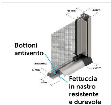
Guida bassa da 17 mm: bottoni antivento e fettuccia in nastro
