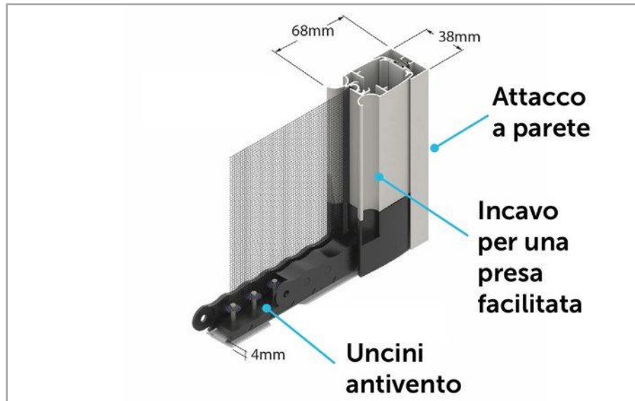
Attacco a parete, incavo per la presa su tutta l'altezza e uncini antivento del «carro armato».
