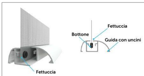
Bottone e fettuccia trattenuti nella guida a uncini
