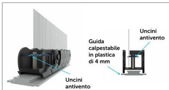
Uncini antivento nel «carro armato», piattina da 4 mm
