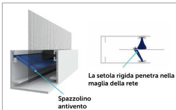
La setola rigida penetra nella maglia della rete
