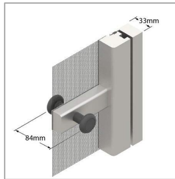
Pomelli interno ed esterno per aprire da entrambi i lati
