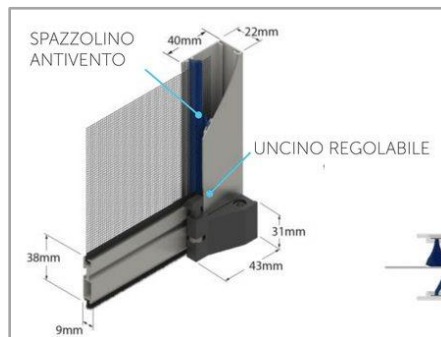
La guida spinge verso l'alto; setole antivento e uncino regolabile
