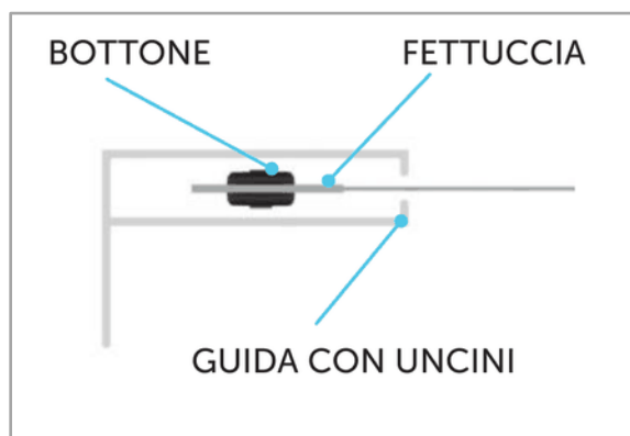
In sezione: bottone e fettuccia nella guida a uncini
