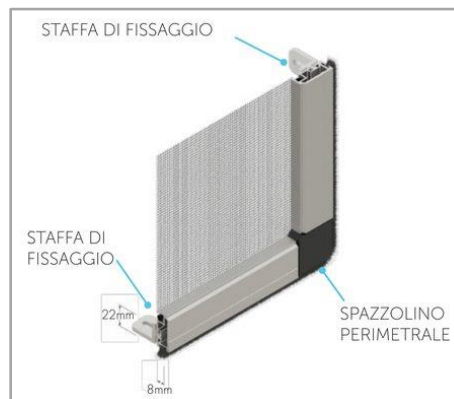
Fissaggio con staffe o con spazzolino perimetrale
