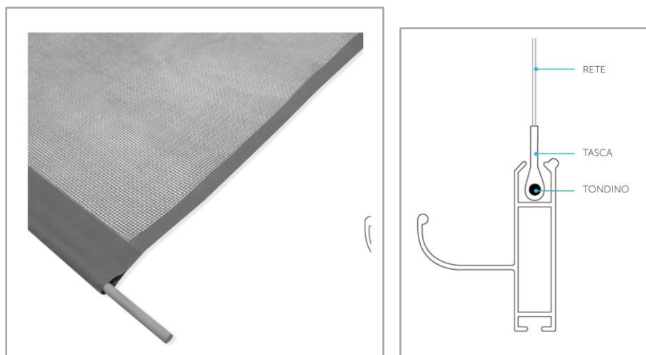
La tasca inferiore con il tondino, vista in sezione.
